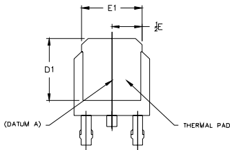
VIEW A-A
